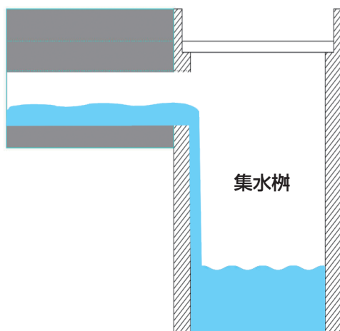
縦断面図
