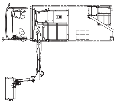
■ イメージ図 上部（作業時）
