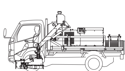
■ イメージ図 後部（作業時）
