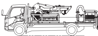
■ イメージ図 上部（作業時）
